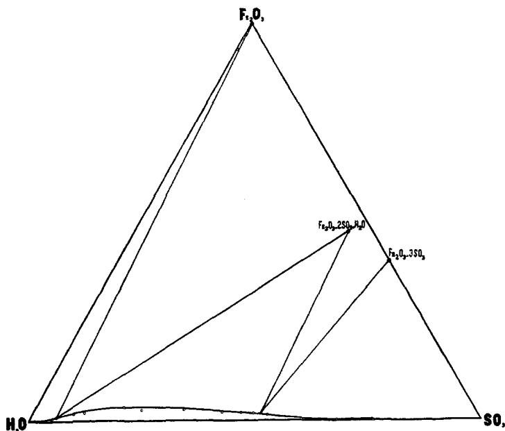
Fig. 4.—200° isotherm.
