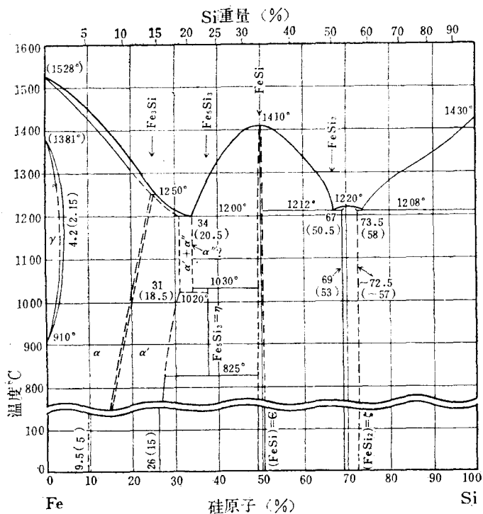
图1 铁-硅系列相平衡图 (根据 Hansen, M (4) .)
