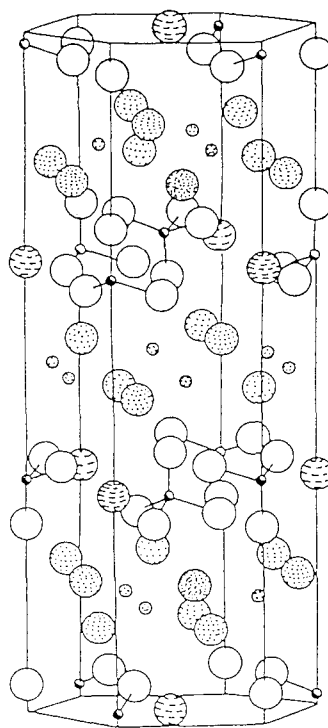
⊖ : M^+ ; ⊙ : Fe^{3+} ; ⊛ : S; ○ : O; ⊕ : OH
