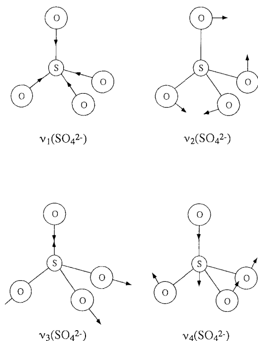
FIG. 8. The \nu_1(\text{SO}_4^{2-}) , \nu_2(\text{SO}_4^{2-}) , \nu_3(\text{SO}_4^{2-}) and \nu_4(\text{SO}_4^{2-}) vibrational modes.
