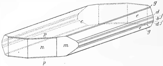
Fig. 4. Epididymite; Narsarsuk.
