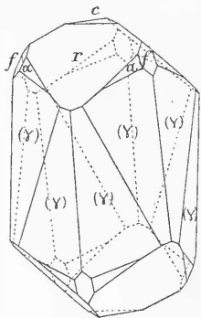
Fig. 1. Calcite; Narsarsuk.
