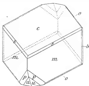
Fig. 10. Neptunite; Narsarsuk.
