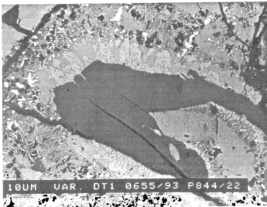
Рис. 1. Подковообразное выделение судовиковита (темная фаза) с коронарным обрамлением фазой PtBiSe (светлое) в клаусталитовой матрице (серое). Изображение получено в режиме детектирования отраженных электронов с помощью полупроводникового детектора. Размер микронного маркера (белый пунктир под кодировочной строкой) указан в начале строки.
