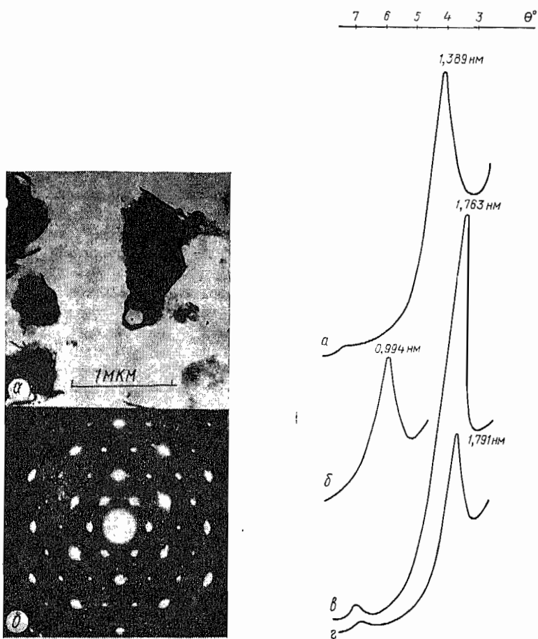
Рис. 1. Электронно-микроскопическое изображение (а) и микродифракционная картина (б) медьсодержащего смектита.
