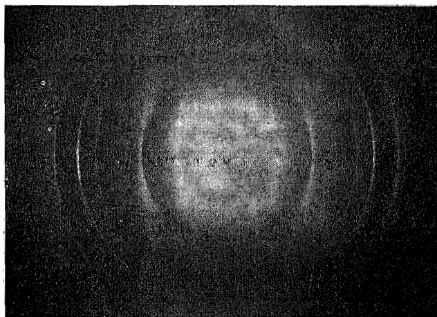
Рис. 3. Электронограмма крестовой текстуры ( \phi=60^\circ ) медьсодержащего смектита.
