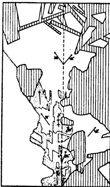
Fig. 3. Durchschnitt eines monoklinen Pyroxens aus dem Eukrit von Juvinas. Das Mineral ist von Anorthit umgeben und im oberen Teil des Bildes von schmalen Leisten dieses Minerals durchschnitten. Der monokline Pyroxen ist im Bilde weiss, der Anorthit vertikal schraffiert. Der Schnitt verläuft nahezu parallel dem Klinopinakoid. Der Pyroxen besteht aus zwei nach 100 verzwillingten Hälften. Die Zwillingsgrenze ist mit --- bezeichnet. Die Felder von schwacher Doppelbrechung in denen eine negative Bisektrix senkrecht austritt sind fein punktiert. Die Pfeile geben die Auslöschungsschiefe c:c in den verschiedenen Teilen des Pyroxens an. Die braunen Felder sind aus der Figur fortgelassen, die orientierten Einschlusstreifen im Pyroxen und die Spaltlinien nach 001 ebenso. Vergr. 33. +
