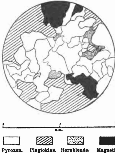
Fig. 2. Parti aus einem Dünnschliff des Diabases aus dem grossen Bergrücken bei Schtschelki. Der grosse „polysomatische“ Pyroxenkomplex ist weiss. Die Grenzen der einzelnen kleinen Körner innerhalb desselben sind durch feine Linien bezeichnet. Die Feldspatfelder sind schraffiert, die einzelnen Plagioklasleisten innerhalb derselben und die kleinen zwischenliegenden Mikropegmatitpartien sind nicht dargestellt. Die Hornblendekörner sind punktiert. Der Magnetit ist schwarz.
