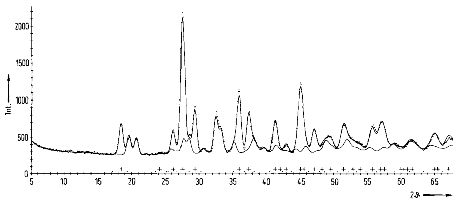
Abb. 3. Neutronenbeugungspulverdiagramm des Gemisches (\text{Fe}_{0,5}\text{Y}_{0,5})(\text{Nb}_{0,75}\text{Ti}_{0,25})_2\text{O}_6 . Die Untergrundlinie enthält neben den (\lambda/2) -Reflexen einer Verbindung mit Rutilstruktur auch die Reflexe einer Verbindung \text{YNbO}_4 mit deformierter Scheelitstruktur
